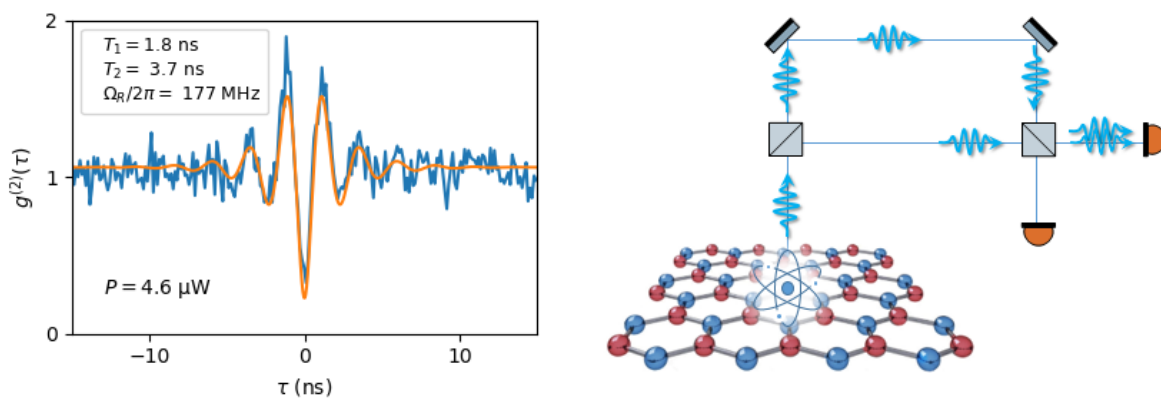
Figure : À gauche, fonction de corrélation de l'émission de photons, qui présente des oscillations qui prouvent la cohérence de l'émetteur. À droite, schéma de l'effet Hong-Ou-Mandel : des photons sont collectés et guidés pour pouvoir interférer.
