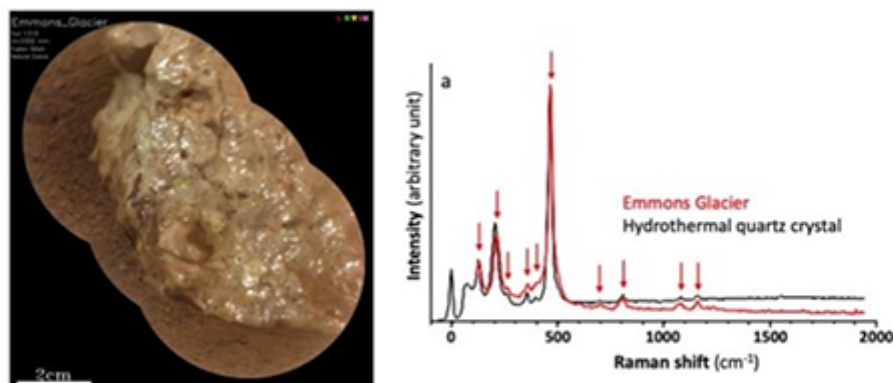
Image obtenue par SuperCam de la roche « Emmons Glacier » (gauche) et Spectre Raman mesuré sur cette cible (en rouge) et comparé à un spectre de quartz hydrothermal mesuré au laboratoire (en noir). Celui-ci indique sans ambiguïté la présence de quartz. Crédits : NASA/JPL-Caltech/LANL/CNES/CNRS
